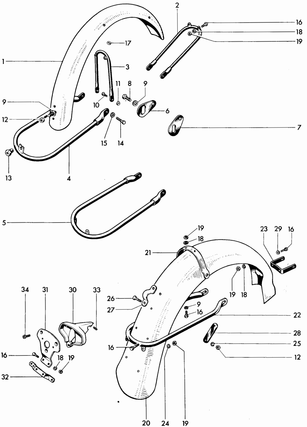
Fig. 23. FENDERS (U.S.A.)
