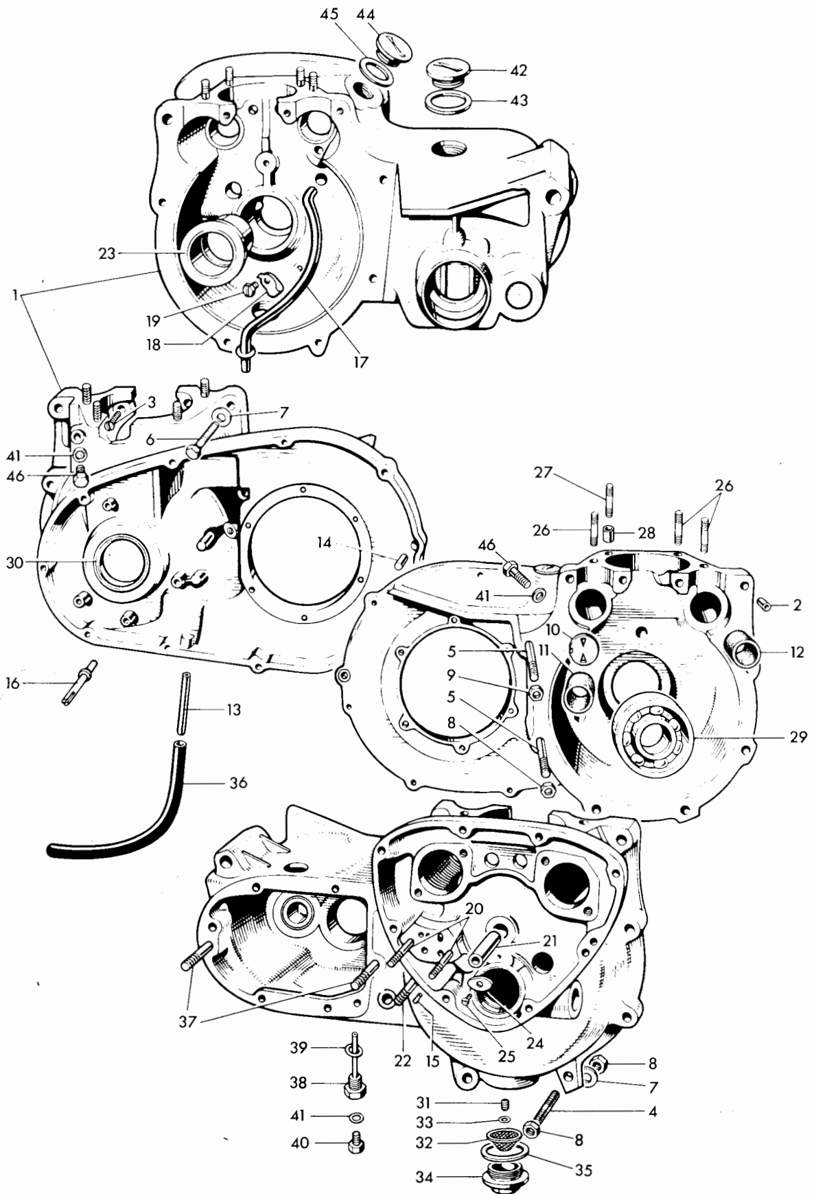
Fig. 2. CRANKCASE
