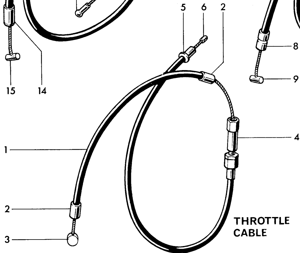
Fig. 29. CONTROL CABLES
